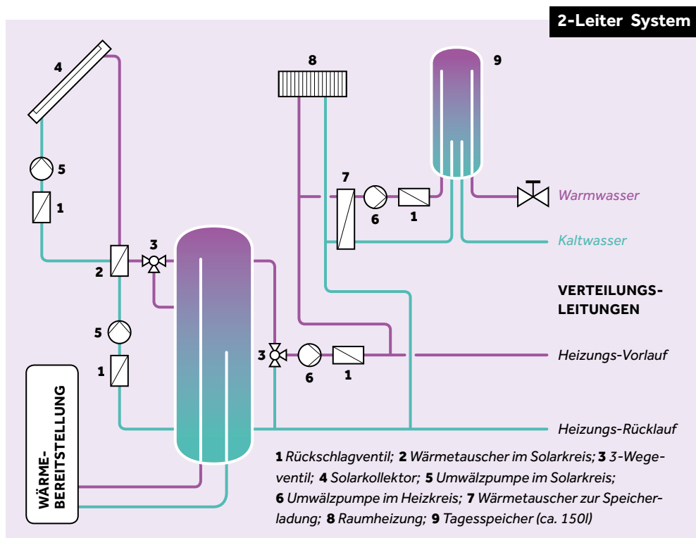
Abb. 5 Schema „Mischform (2-Leiter-System)“ Quelle: ALLPLAN
