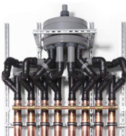
Abb. 20 Zentraler Gegenstrom-Wärmetauscher Quelle: Fa. Hei-Tech
