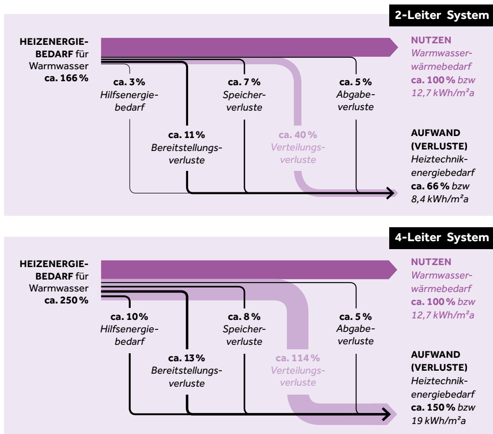
Abb. 7 Energieströme bei der Warmwasserbereitung: Größenordnungen für 2-Leiter- (oben) und 4-Leiter- (unten) System, 20 Wohnungen Quelle: ALLPLAN 15
