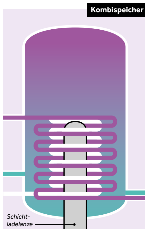
Abb. 12 Aufbau eines Kombispeichers mit Wellenrohr-Wärmetauscher Solarfocus GmbH, 2015
