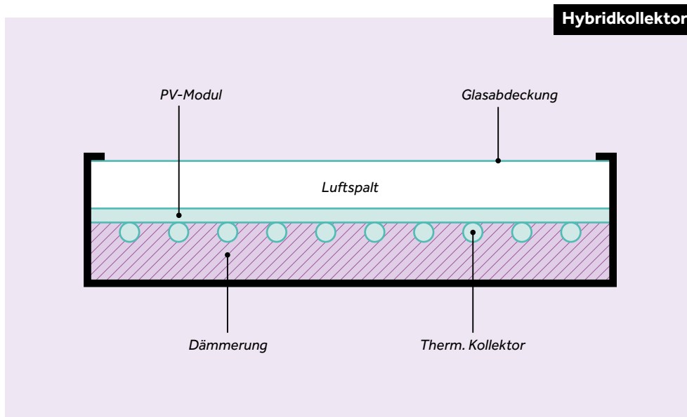
Abb. 25 Wassergekühlter abgedeckter Hybridkollektor Quelle: ALLPLAN
